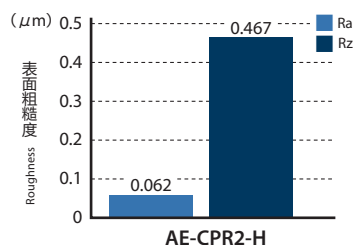
平面部的表面粗糙度
